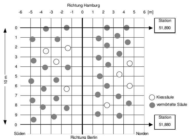
Bild 11: Ausschnitt aus der Dokumentation des Säulennasters bei -2,7 m unter SO als Entscheidungsgrundlage für die Herstellung des Tragsystems
