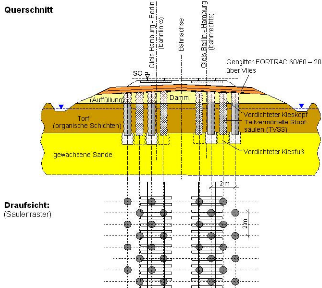
Bild 2: Querschnitt und Draufsicht nach der 1. Ausbaustufe
